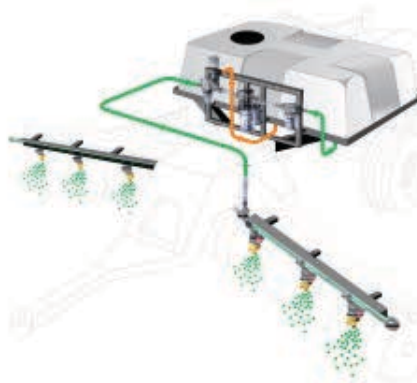
Tárcsára szerelt szórófej sor
